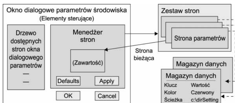
Rysunek 11.3. Struktura okienka parametrów systemu i zawartej w nim strony
