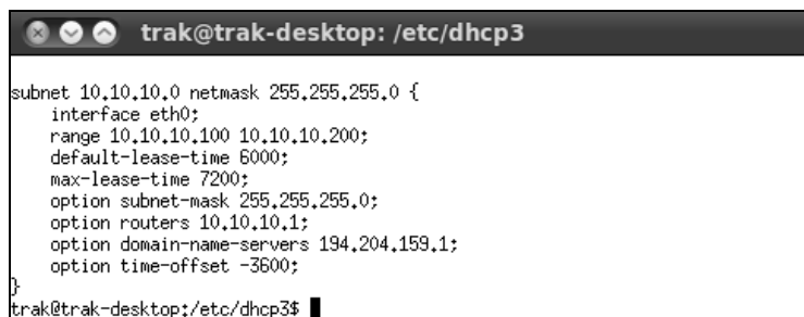
Rysunek 2.23. DHCP: a) zawartość pliku konfiguracyjnego dhcpd.conf ,
