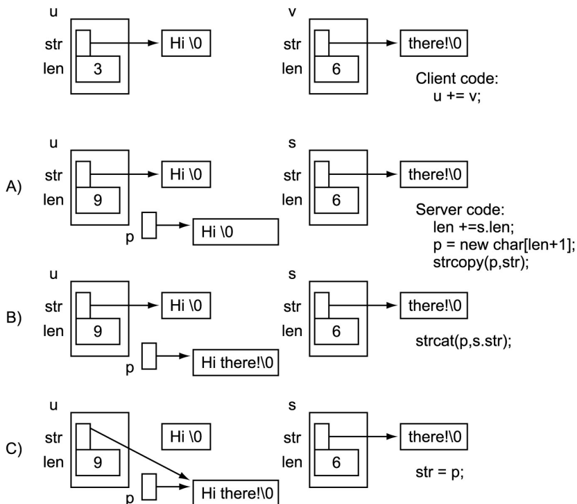
Rysunek 11.7. Schemat pamięci dla funkcji operatorowej konkatenacji łańcuchów znakowych
