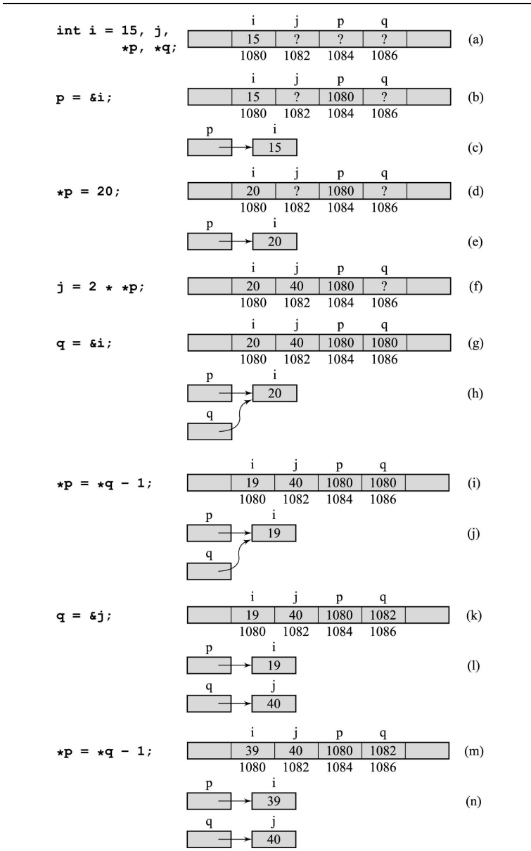
RYSUNEK 1.1. Zmiany wartości po przypisaniach realizowane są przy użyciu wskaźników. Przypadki (b) i (c) opisują tę samą sytuację, tak samo (d) i (e), (g) i (h), (i) i (j), (k) i (l) oraz (m) i (n)
