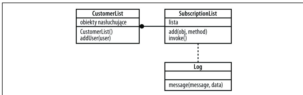
Rysunek 7.1. Obiekty CustomerList oraz związany z nim obiekt SubscriptionList wraz z obiektem Log
